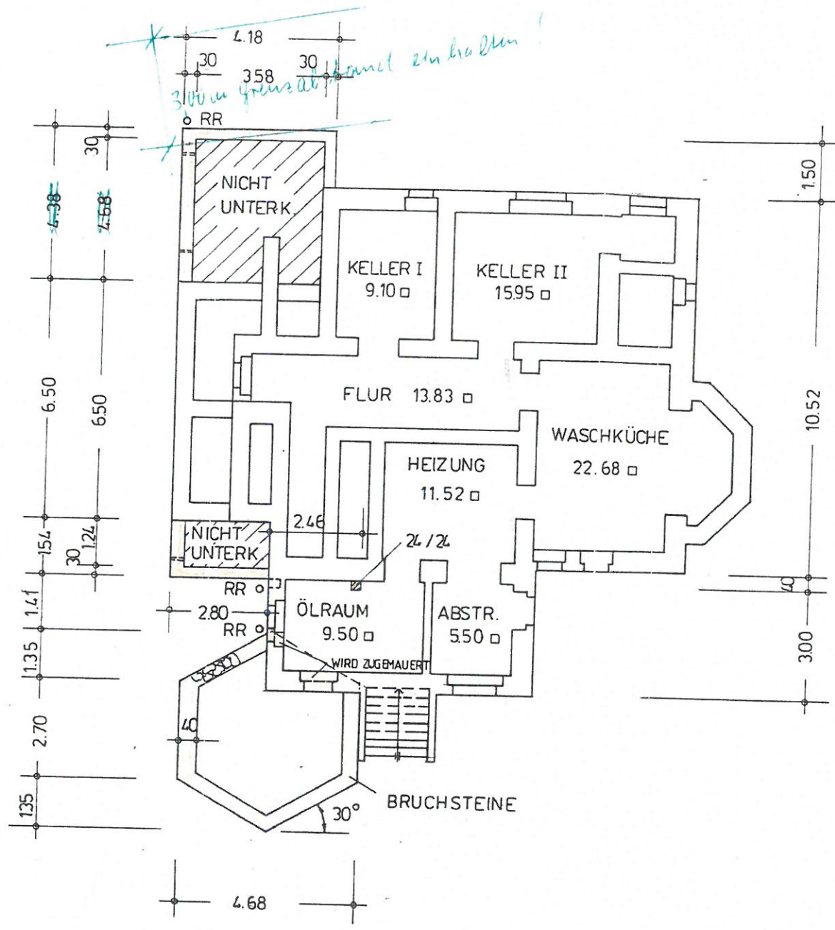
KELLERGESCHOSSGRUNDRISS
