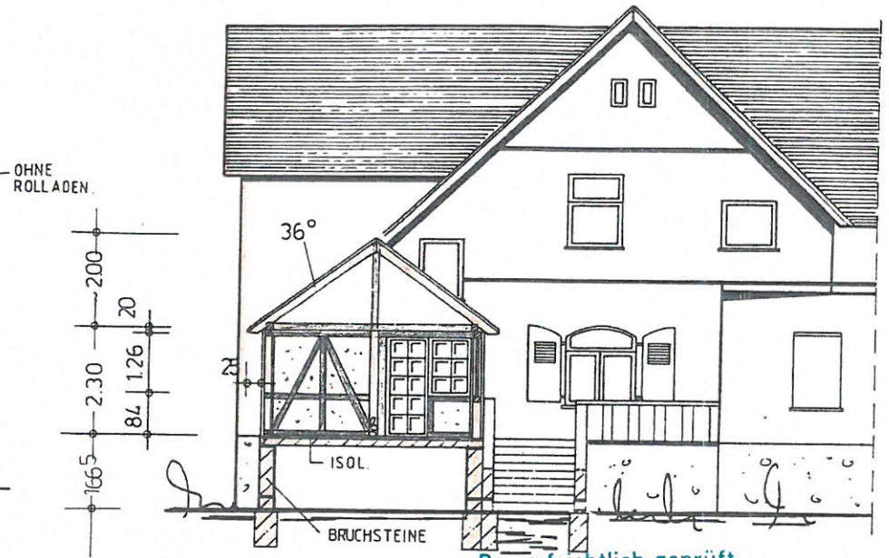
SCHNITT: b-b
